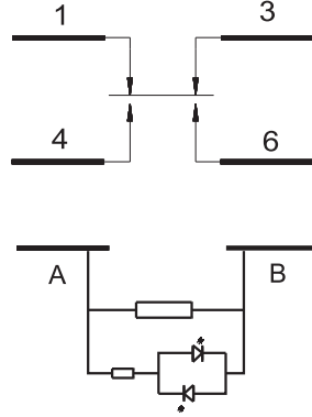
QZ(HF10FF-Q/HF10FF-QV/HF10FH-Q/HF10FH-QV 带发光二极管)
