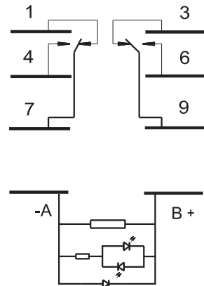
2Z(HF10FF-Q/HF10FF-QV/HF10FH-Q/HF10FH-QV 带发光二极管和续流二极管)
