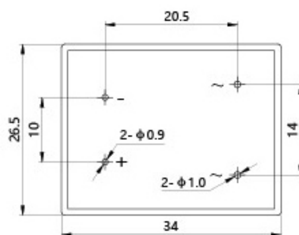
安装尺寸
