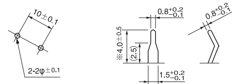
(基板孔尺寸)
